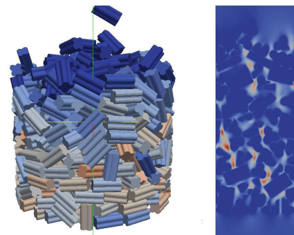
Simulation d'un écoulement en réacteur à lit fixe : empilement de catalyseurs (gauche) et champ de vitesse (droite).
