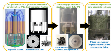
Réacteur agité triphasique : de la CFD (gauche) à la réalité technologique (droite).
