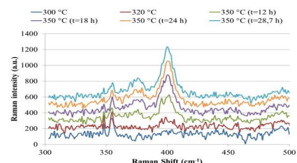
Suivi temporel de la phase active ( \text{MoS}_2 à 375 et 400 \text{ cm}^{-1} ) lors de l'activation d'un catalyseur CoMoP.
