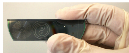
Puce microfluidique pour l'acquisition de données thermodynamiques.
